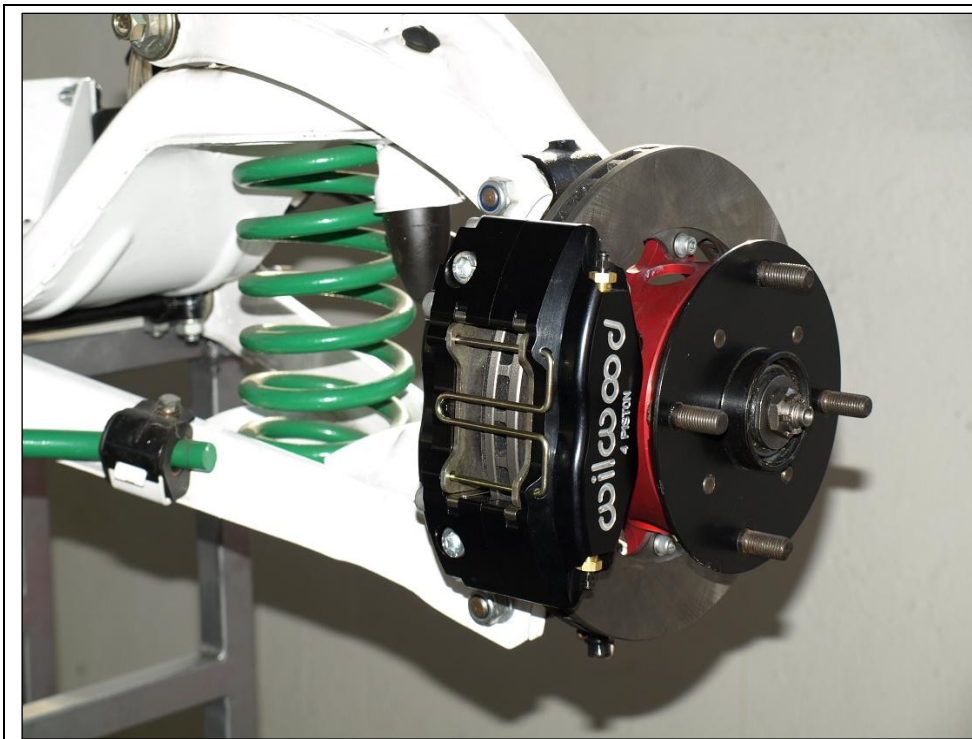
Kompletace na nápravě – provedení s chlazeným kotoučem.
