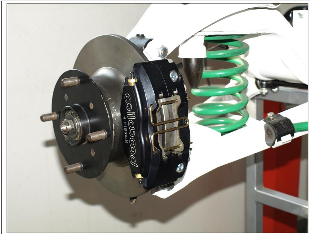
Kompletace na nápravě – provedení s plným brzdovým kotoučem.
